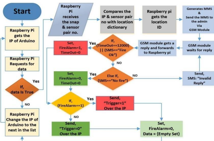
Fig.3.LogicdiagramofcontrollingofRaspberryPi.
