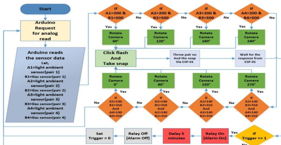
Fig.4.LogicdiagramofoperationofArduino.
